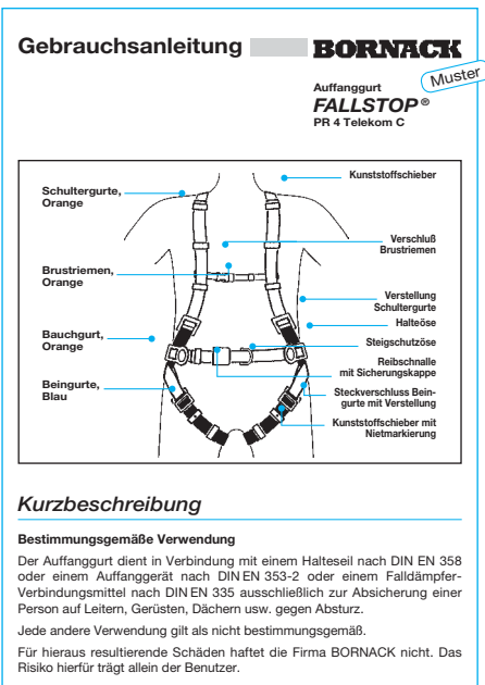
Bild 1-5: Muster einer Gebrauchsanleitung (siehe Anhang 4)
