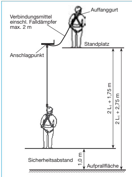
Bild 2-13: Freiraum unterhalb des Benutzers
