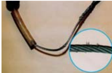
Bild 5-8: Schadhafte Verbindungsmittel
